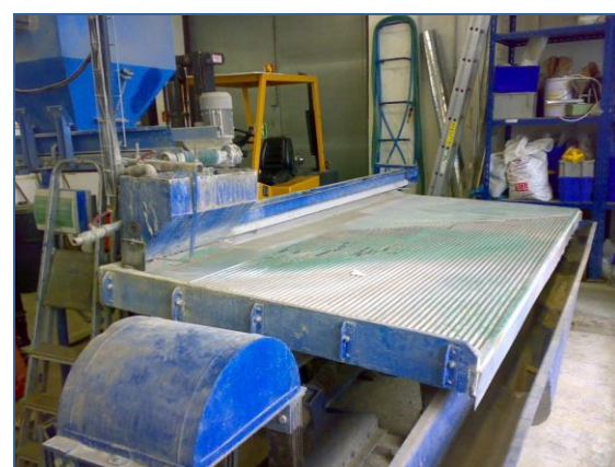
Mokrý gravitační splav
